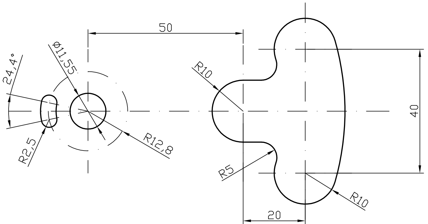
Dettaglio "A" SCALA 1:1
